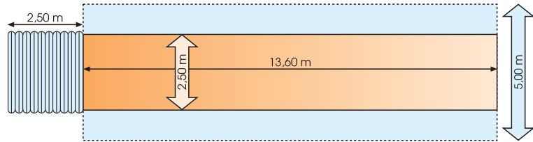
Schiebebügelaufleger - freier Zugang zur Ware, 2,84 m Ladehöhe, 27 t NL
