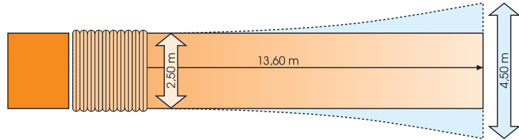
Rechter Dachgurt nach innen - links verschoben - von rechts frei beladbar
